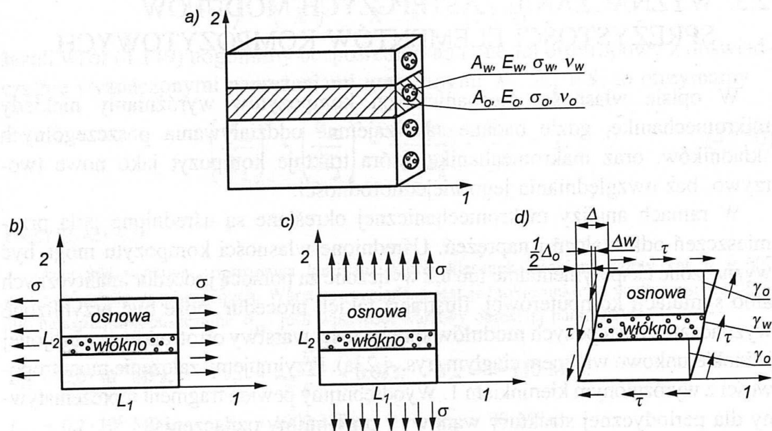
Modele obciążeń powtarzalnego segmentu kompozytu z włóknem ciągłym stosowane do wyznaczenia zastępczych stałych sprężystych
