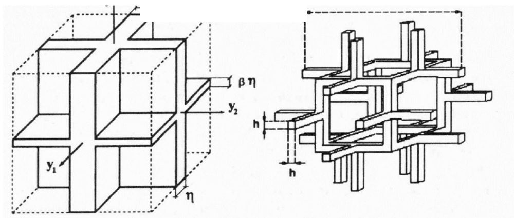
a) model do analitycznej homogenizacji periodycznej struktury porowatej
